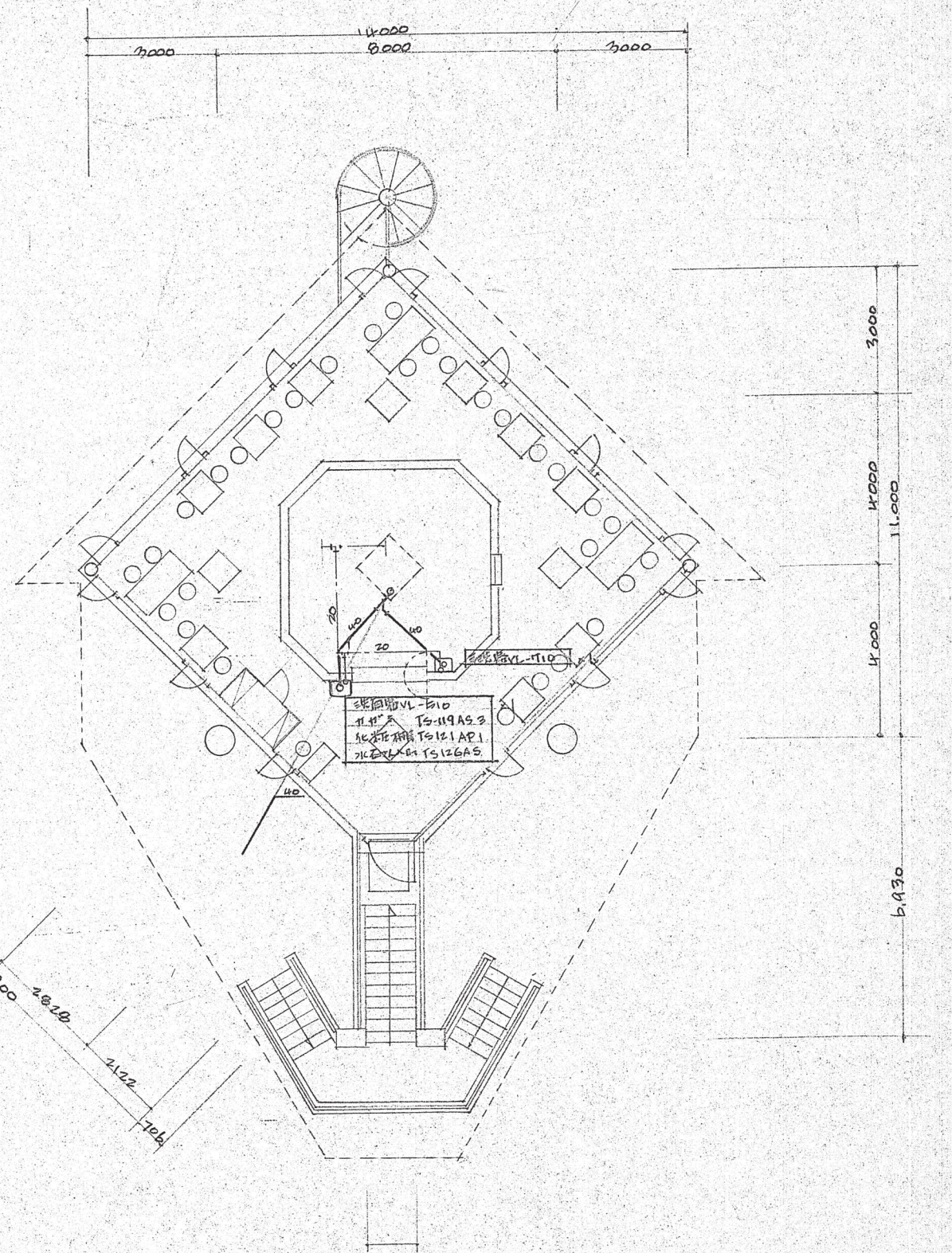
2階 平面圖 1:100
