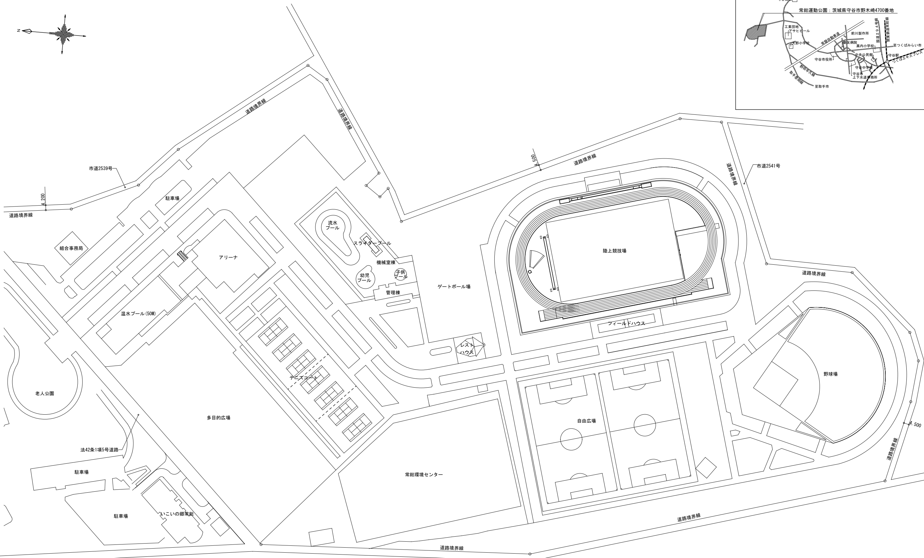
公園全体配置図 NON SCALE
